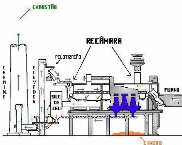
Desenho n.º 1 – Recâmara de forno ACL da Allis Chalmers
