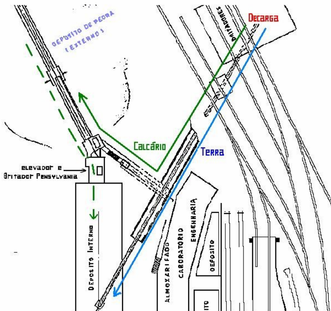
Desenho n. ° 3 - Entrada de matéria-prima
